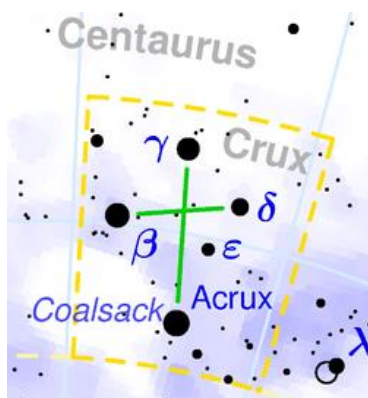
Suhvězdí Jižní kříž
